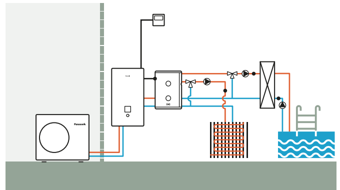
Aquarea J- und H-Generation: Zwei Heizkreise mit Aquarea Splitsystem, Pufferspeicher und Schwimmbadheizung
