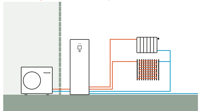
Aquarea J- und H-Generation: Zwei Heizkreise mit Aquarea Kombi-Hydromodul in Ausführung „B“ 1 , ohne Pufferspeicher
