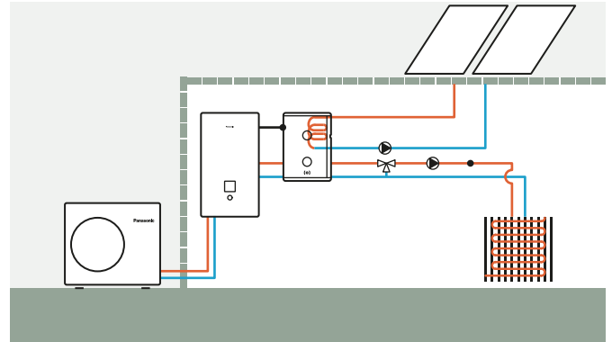
Aquarea J- und H-Generation: Heizungssystem mit Aquarea Splitsystem, Pufferspeicher, Solarthermieanlage und Mischventil
